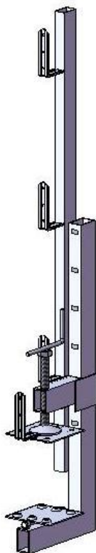
11_77_Aggancio Superficie orizzontale
